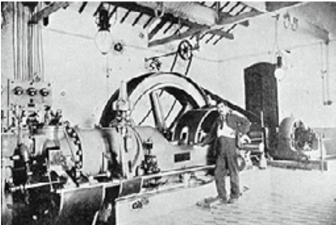
Motor de gas pobre para accionar las motobombas de elevación de agua.
